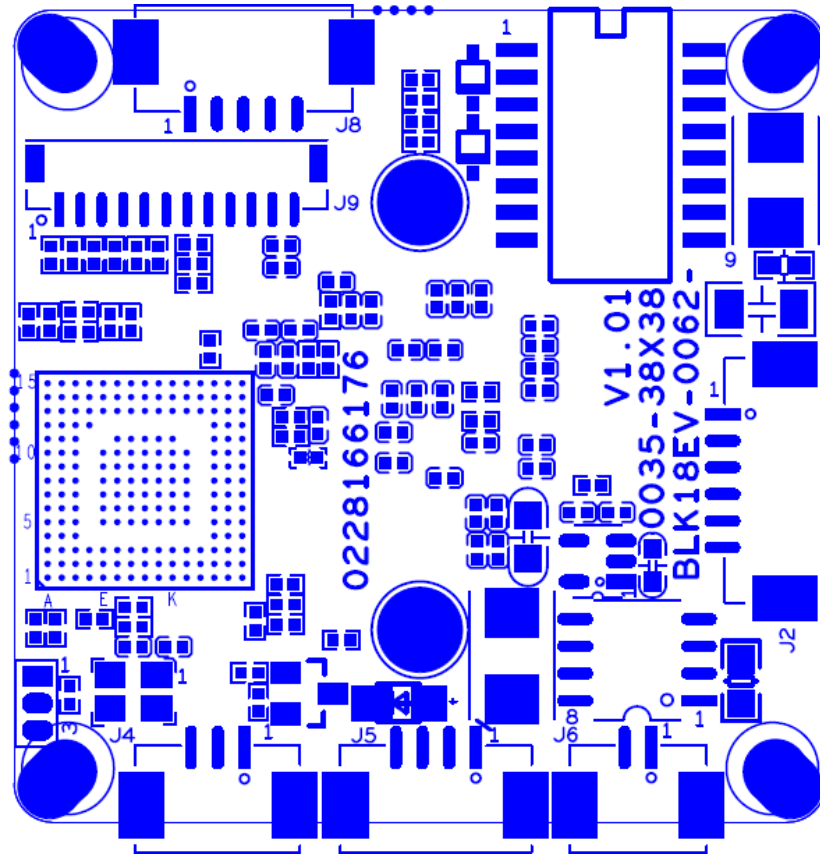
BLK18EV-0062-0035-38X38-V1_01 Interface Description
