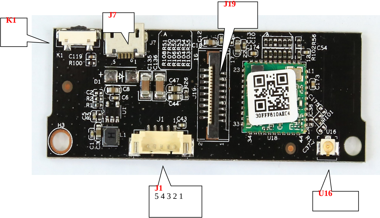
IPC-RM510-WIFI-USB-IF-S-V2_01 接口说明
