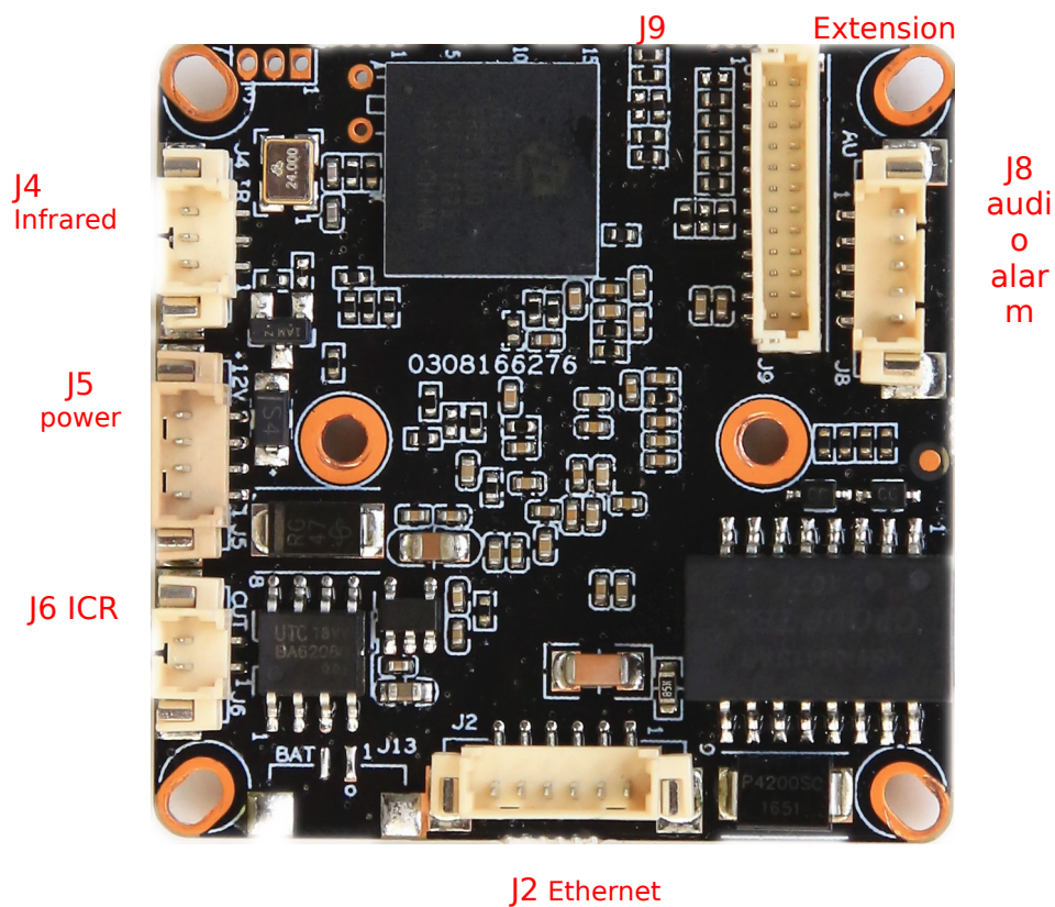
BLK18EV-0065-0130-RTC-38X38-V1_01 Interface Description
